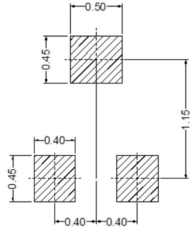
SOT-723
