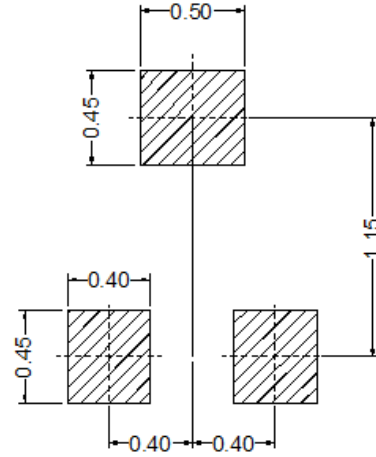
SOT-723
