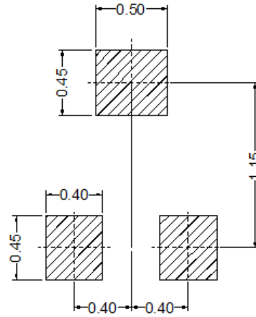
SOT-723
