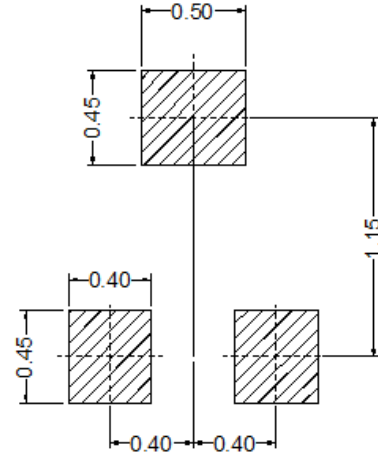
SOT-723
