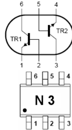
SOT-363
