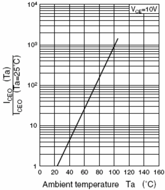
I_{CEO} - T_a
