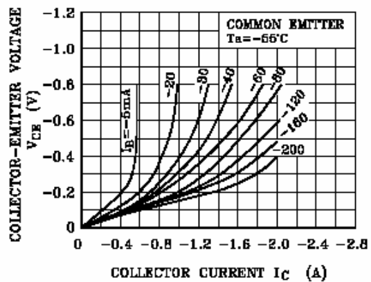
V_{CE} - I_C
