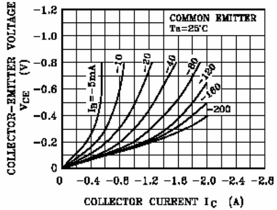
V_{CE} - I_C
